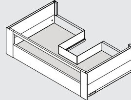
EY/Z boxcover - galerie
