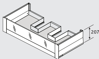
EY2/Z boxcap - verre haut
