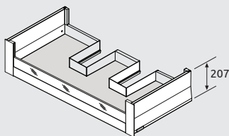
EY2/Z boxcap - verre bas
