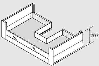
EY/Z boxcover - verre bas
