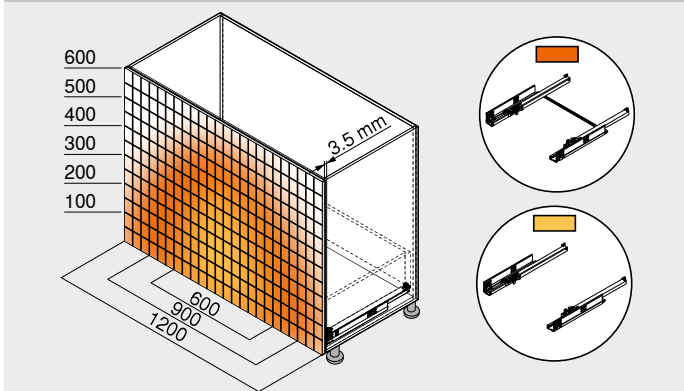
Exemple pour 560H – 30 kg, longueur nominale NL 500 mm, tiroir à quatre côtés, avec synchronisation
