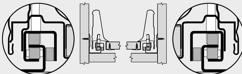
Compensation totale des tolérances \pm 1.5 mm dans le système
