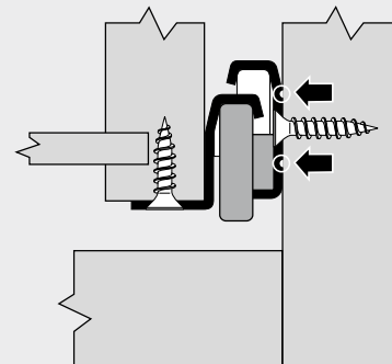
Deux emboutissages évitent un éventuel frottement sur des têtes de vis saillantes
