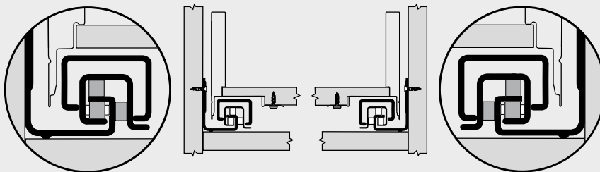
Compensation totale des tolérances \pm 1.5 mm dans le système
