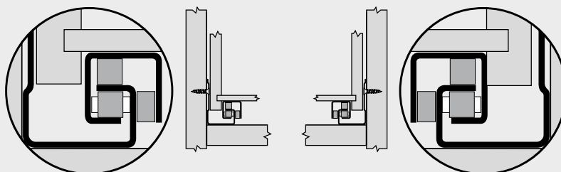
A gauche, compensation totale des tolérances +1.5 / -0 mm 1
